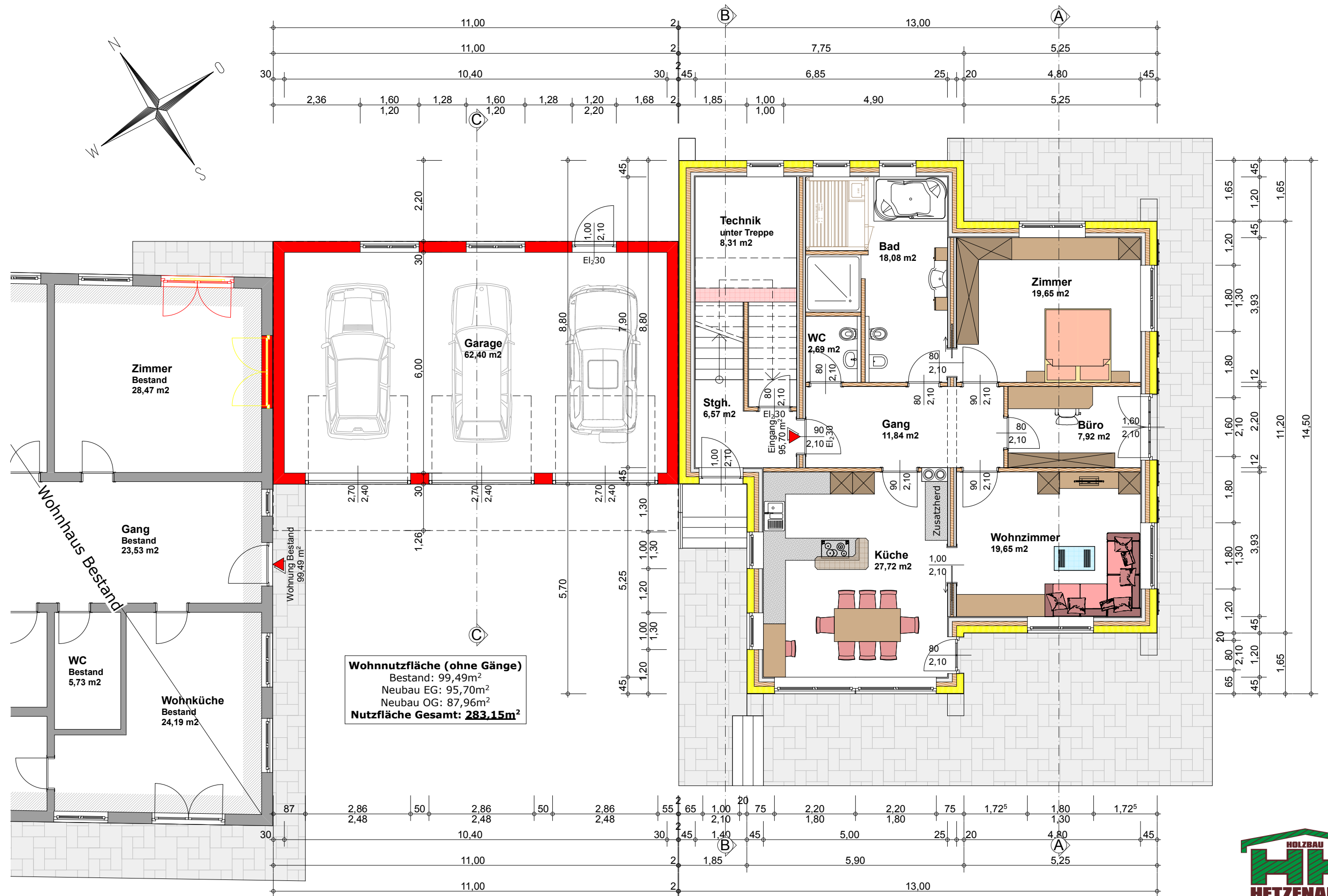
Neubau eines Einfamilienhauses Grundriss Erdgeschoss (M 1:100)
